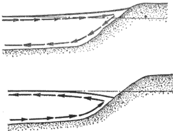
Рис.: схема образования прибрежных течений при морской бризе (верхний рисунок) и при береговом бризе.
